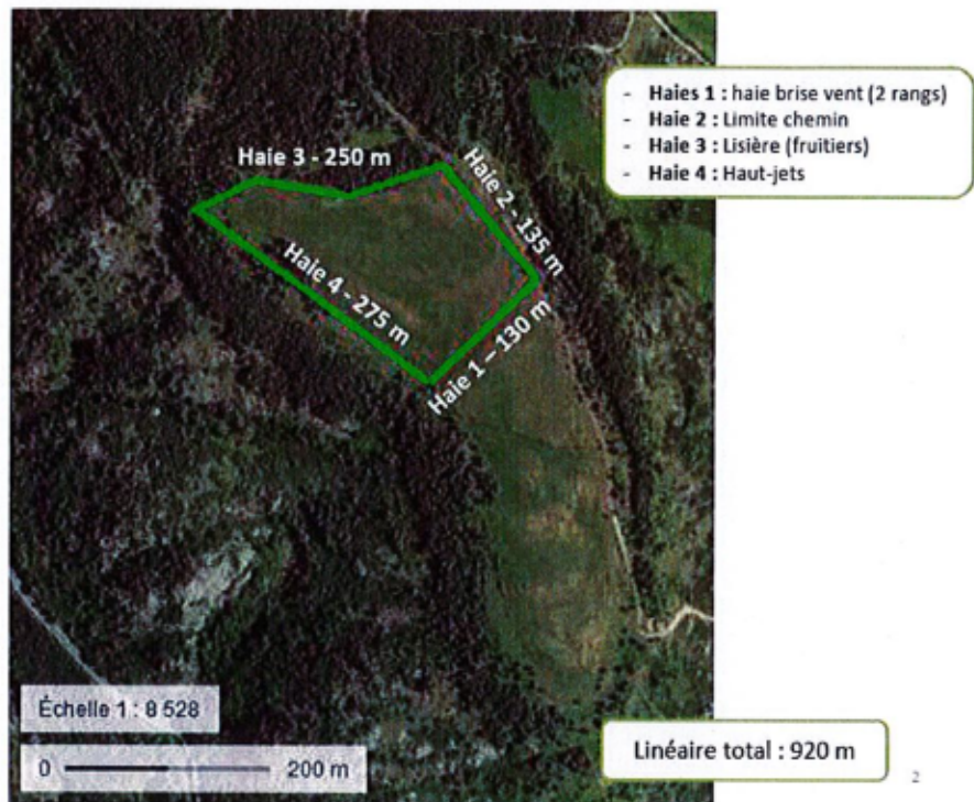
Extrait du plan d'aménagement 48 Causse_Marazeil
