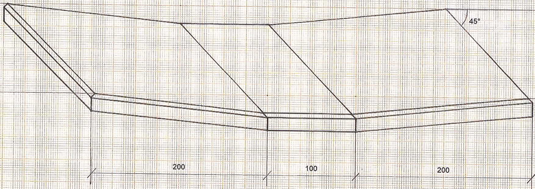
Coupe-eau béton (échelle 1/25 + détail 1/5)
